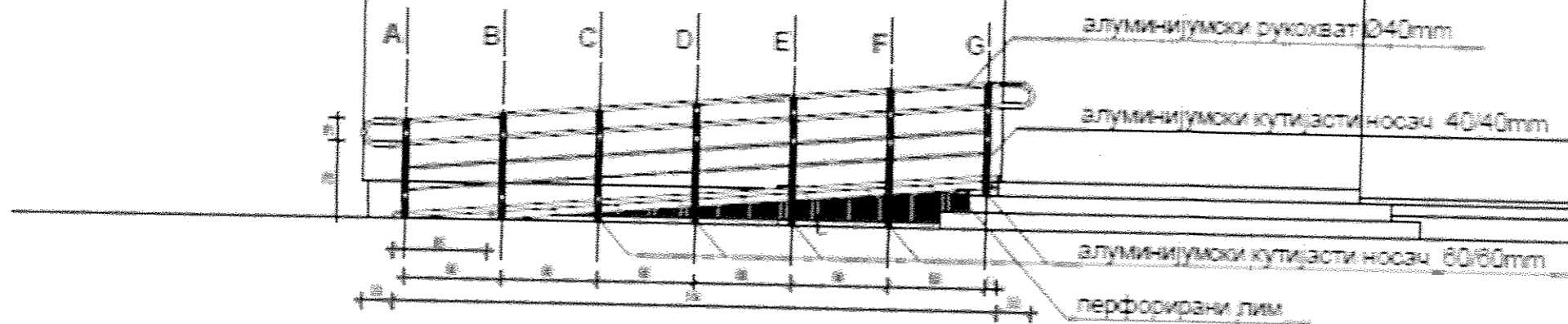
ИЗГЛЕД РАМПЕ
